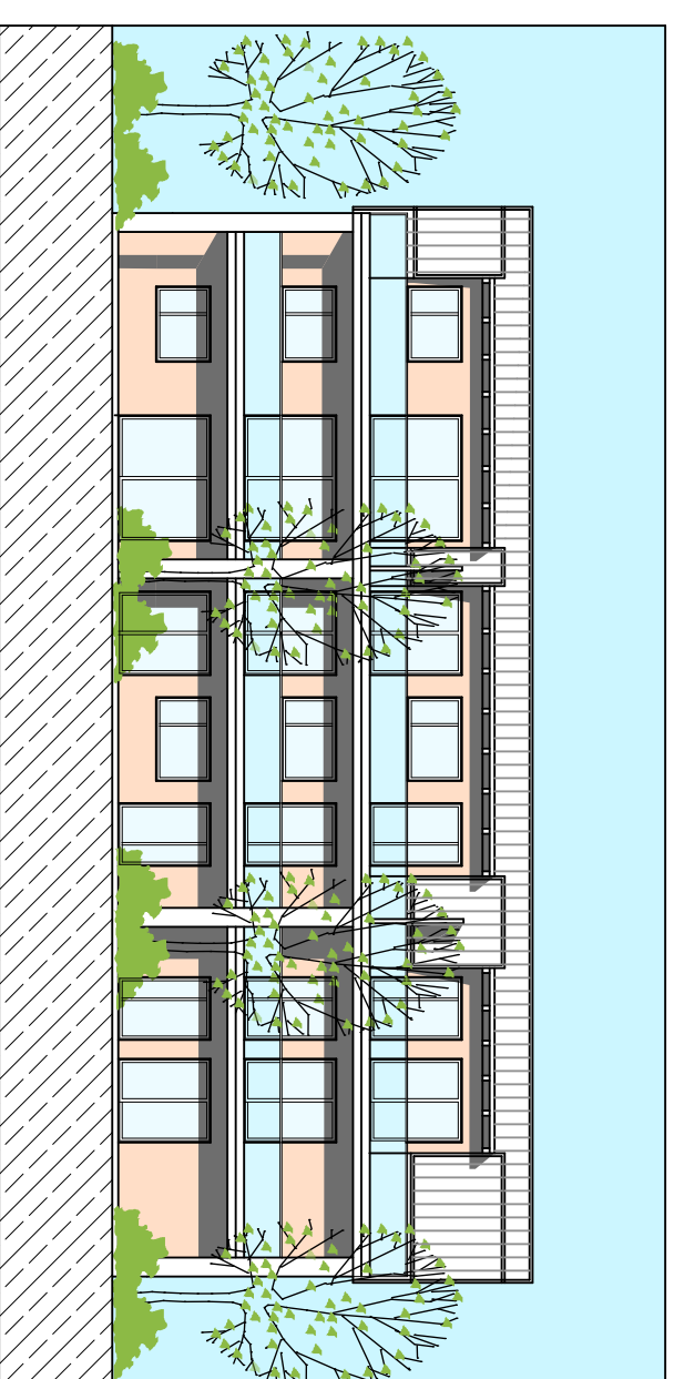
SÜDANSICHT
